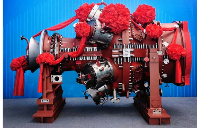
◀ 国内首台自主研发 15 兆瓦重型燃气轮机
